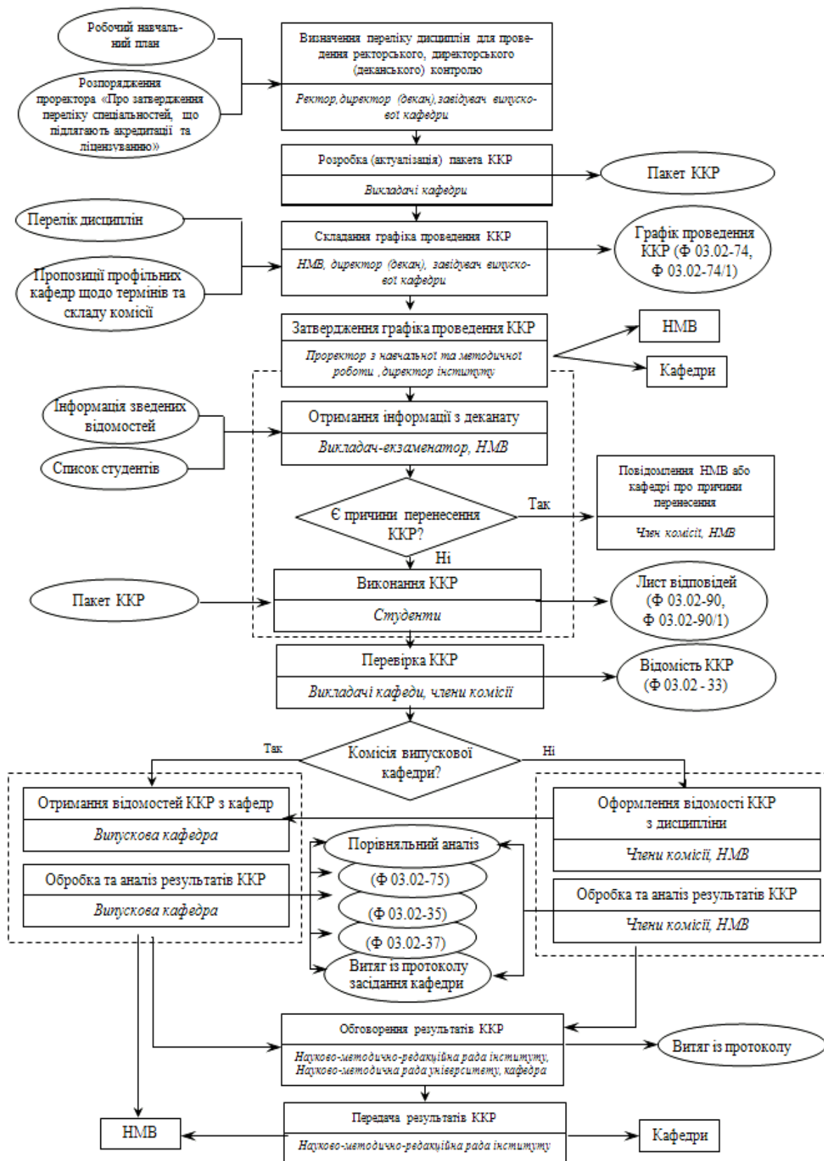
Рис 1. Алгоритм підготовки, проведення та аналізу результатів ККР
